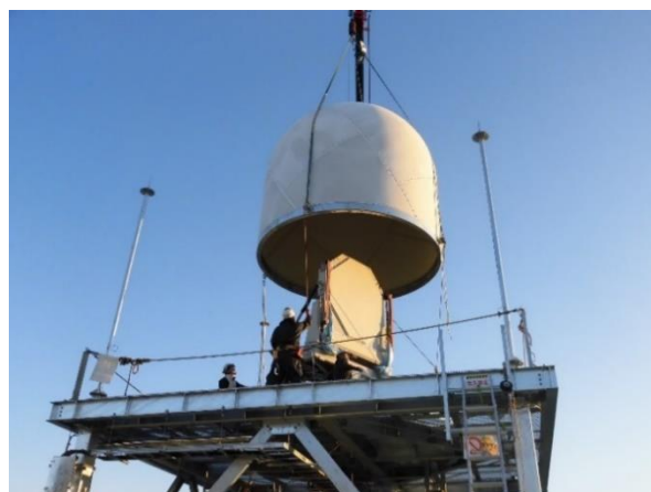
MP-PAWR 埼玉大学設置時の様子 (アンテナにレドームを被せる直前)
