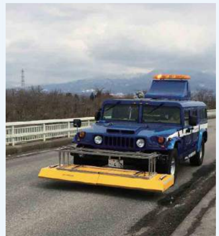
車載型高速スキャンレーダーによる床版内部の診断
