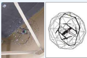
受動回転球殻マルチコプタ
