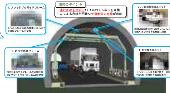
トンネル全断面点検・診断システム
