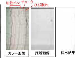
取得画像とひび割れ検出結果
