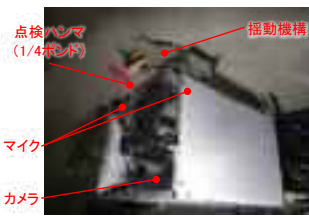
打音検査ユニット
