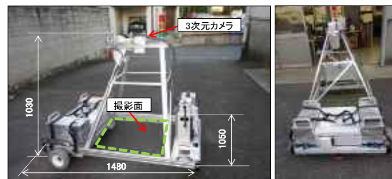
全方位型ロボット(側面)
