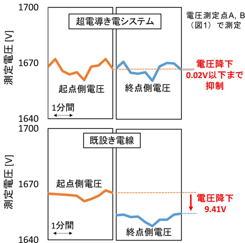
図2 超電導き電による電圧降下の比較
