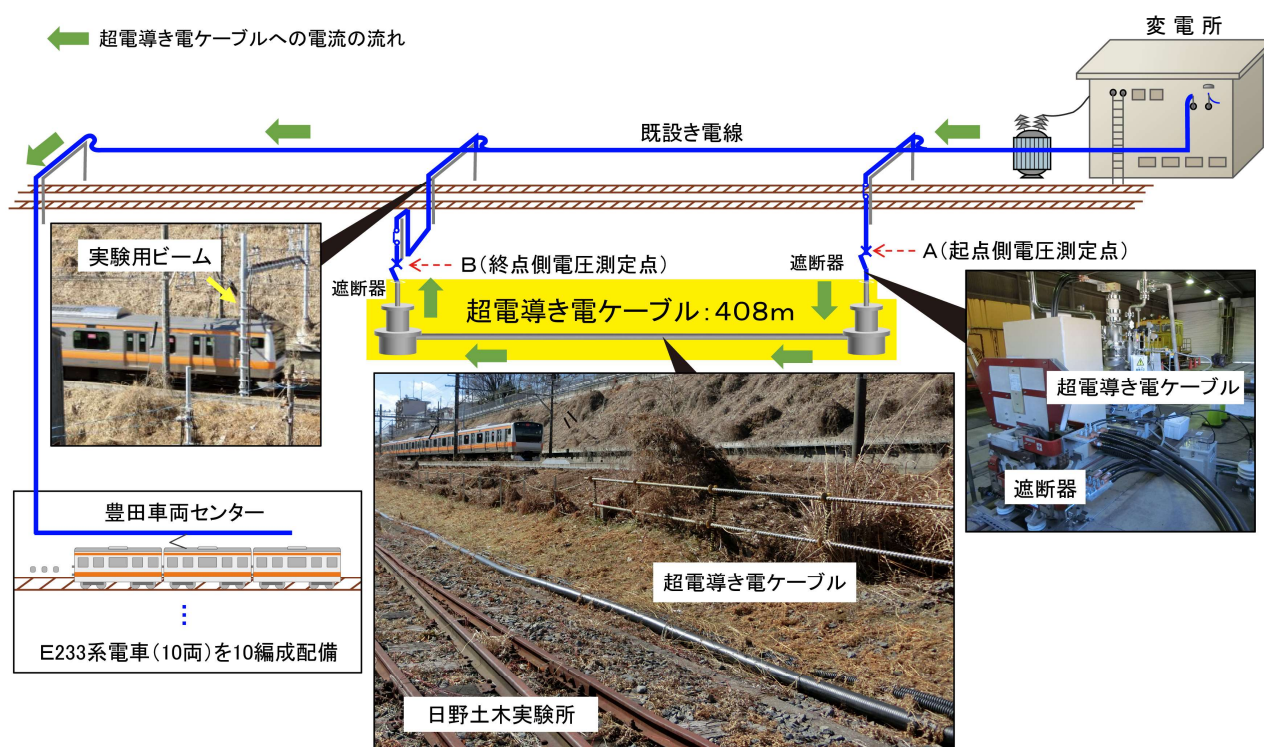
図1 試験時の送電設備と超電導き電ケーブルへの電流の流れ
