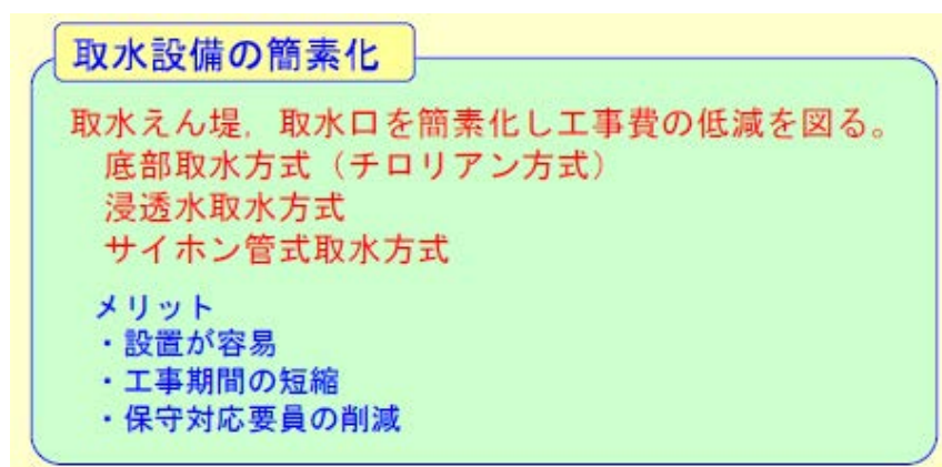
図 26 取水設備の簡素化技術
