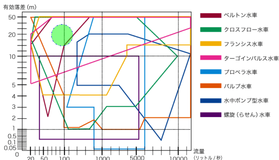
図 33 水車選定図
