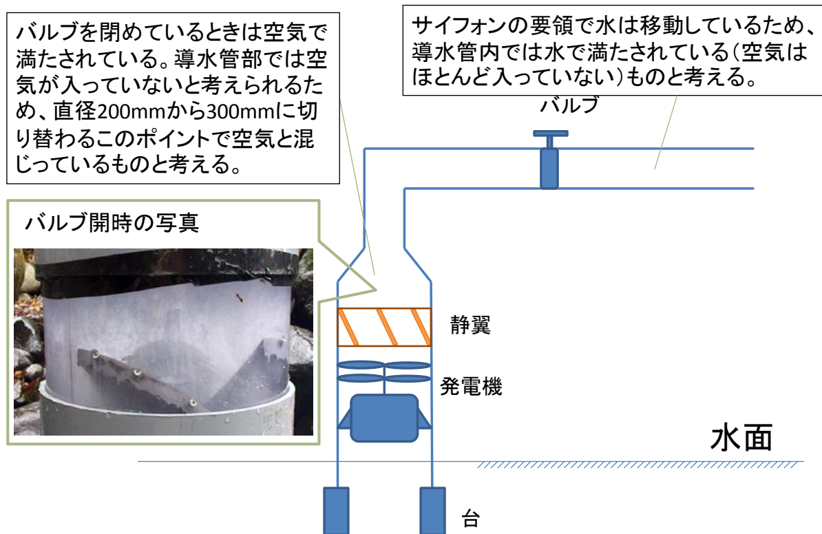
図 44 発電装置の全体図
