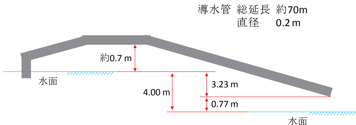
図 41 導水管全体図
