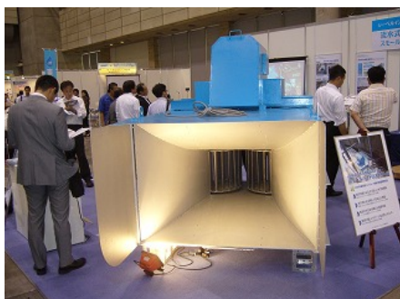
図 29 スモールハイドロストリーム (再生可能エネルギー世界フェア 2010 にて撮影)
