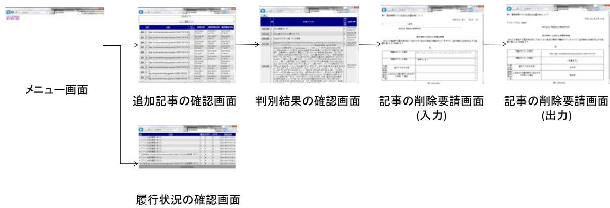
図 41 画面遷移図
