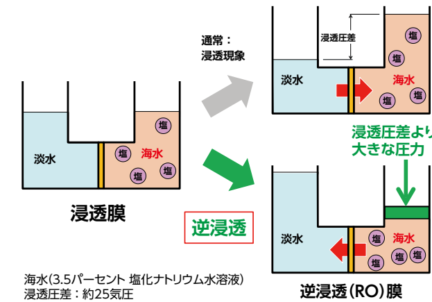
■図2 直径約0.5ナノメートル(ナノは10億分の1)の孔が無数に開いた膜は、水分子だけを通して不純物を通さない。この膜を隔てた左右にそれぞれ淡水と海水を入れたら、同じ濃度になるように淡水側の水分子が海水側へ流入する。この時、膜には濃度に応じた浸透圧が発生するが、それよりも大きい圧力を海水側にかけることで、海水の水分子だけが膜を通して淡水側へ移動する現象が「逆浸透」である。
