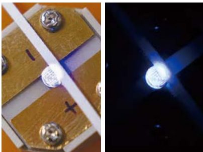
■図4 270ナノメートルの深紫外線を発生する深紫外LED。2014年には殺菌用途で市販化された。
