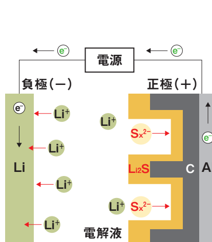
正極に硫黄+炭素、負極にリチウム、電解質にイオン液体を積み重ねて作られた試験用のセル（ボタン電池）。
