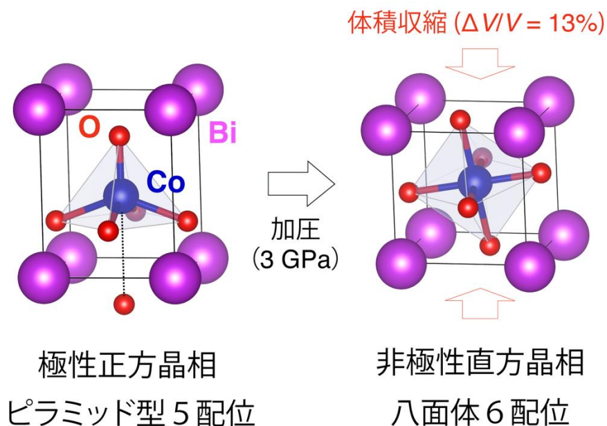
図 1: コバルト酸ビスマス \text{BiCoO}_3 の圧力下での結晶構造の変化。CoO 5 ピラミッド型 5 配位の極性正方晶構造から、CoO 6 八面体 6 配位の非極性直方晶構造への構造相転移により、13%の巨大体積収縮が生じる。
