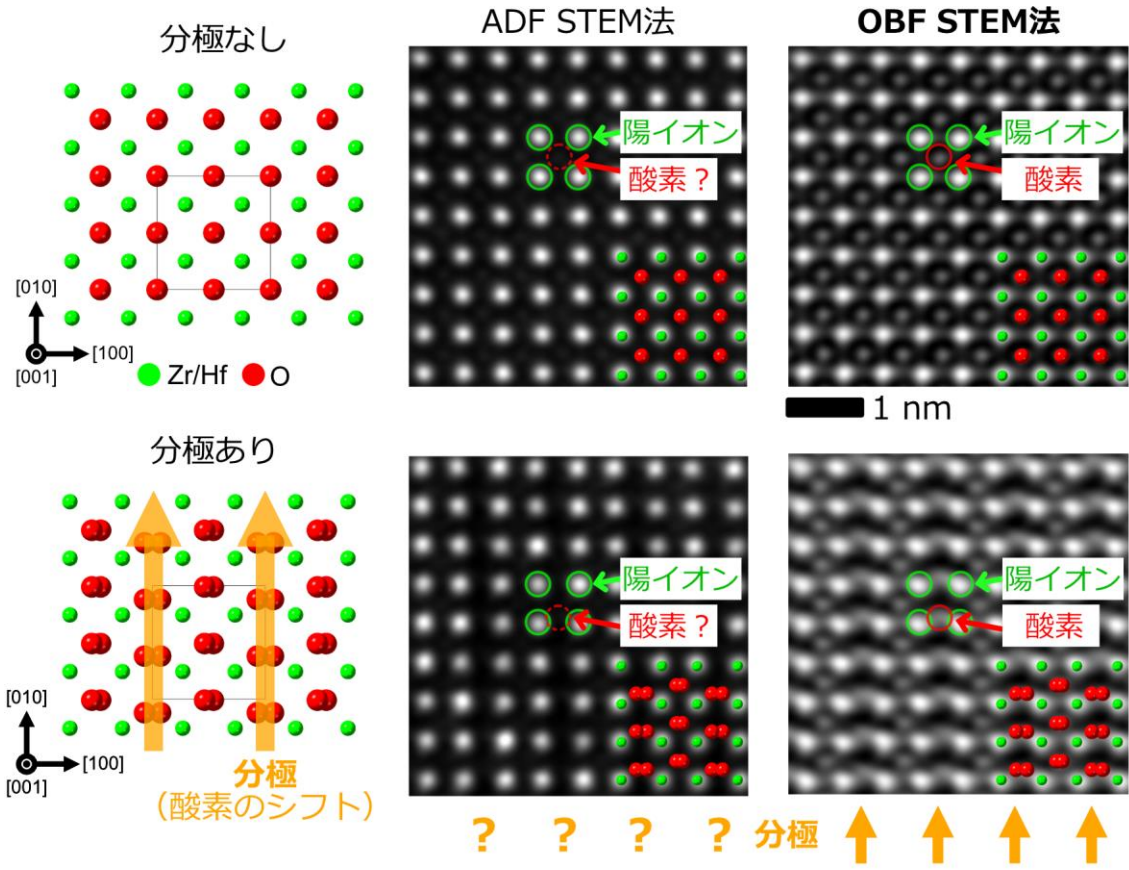
図2 蛍石型強誘電体の分極の有無に応じた原子構造と ADF STEM 像ならびに OBF STEM 像
