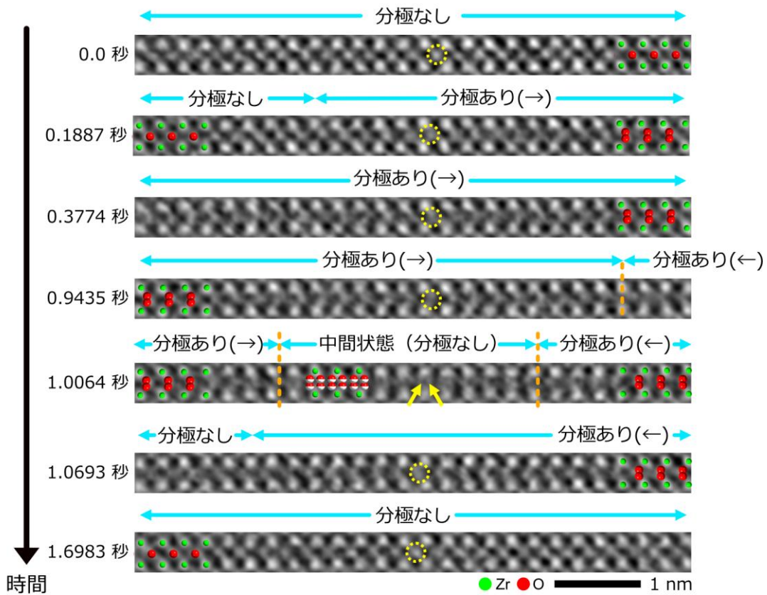
図3 高速スキャンOBF STEM法によって捉えた分極反転における原子の動きのその場観察
