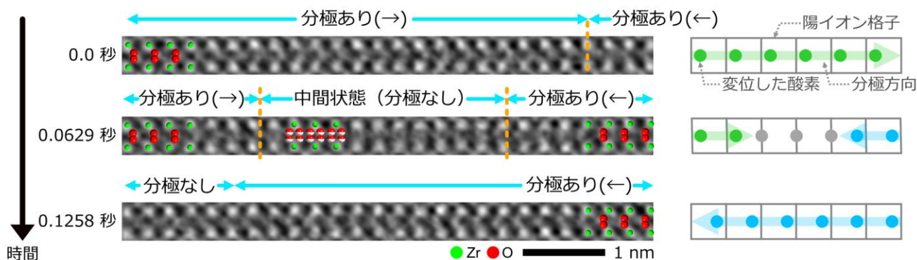
図1 蛍石型強誘電体にて直接観察された分極反転中の原子の動き
