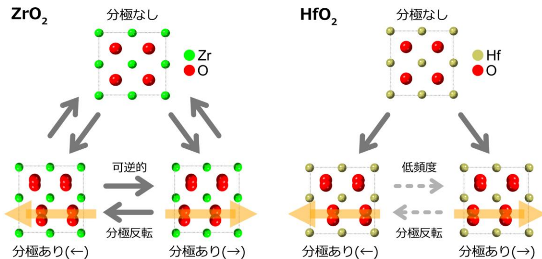
図4 第一原理計算によって検証された ZrO_2 および HfO_2 における分極反転の起こりやすさ
