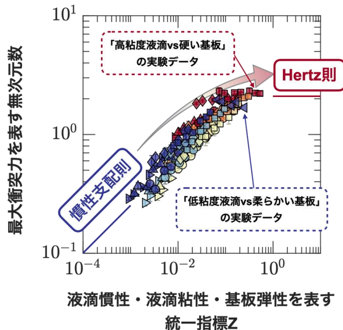
図 2 統一指標 Z を用いた最大衝突力のスケージング則の移行：多数の実験条件で得られた最大衝突力のデータが、液滴粘性・液滴慣性・基板弾性を包含する統一指標 Z を用いることで慣性支配則から Hertz 則への連続的な移行を、1つの法則（マスターカーブ）で理解できる。「低粘度液滴が柔らかい基板上に衝突する場合」が「高粘度液滴が硬い基板に衝突する場合」と同様の振る舞いを示している。（Yokoyama et al. , Nature Communications, 2025 を基に作成）
