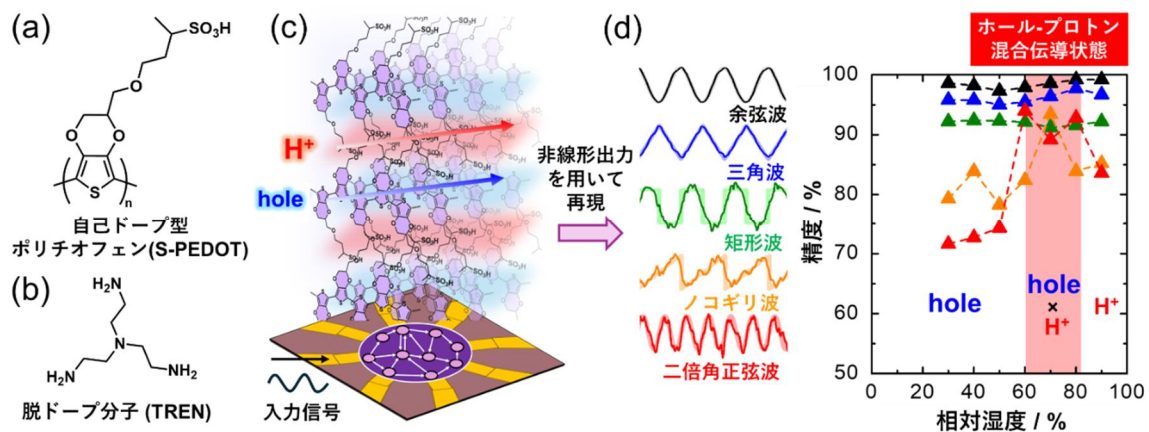
図 1. (a) 自己ドーブ型ポリチオフェン (S-PEDOT) と (b) 脱ドーブ分子である多価アミンの化学構造、 (c) 本系におけるホール-プロトン混合伝導状態を示すイメージ図。(d) 混合伝導状態を示す条件にて マテリアリザバー素子の性能 (波形生成タスクの精度) が向上することを示す図。
