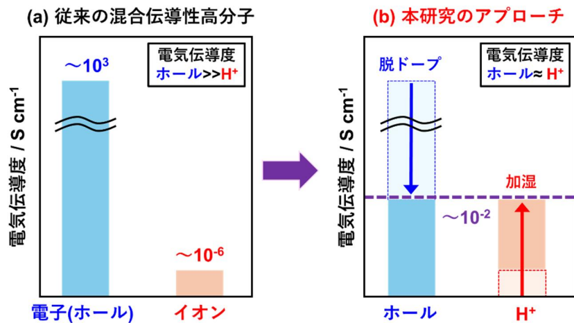
図 2. (a) 従来の混合伝導性高分子における電子（ホール）とイオン（プロトン）の電気伝導度を比較した図。イオン伝導度は電子伝導度と比較して圧倒的に低いため、主要な伝導キャリアは電子となっている。(b) 本研究のアプローチで実証したホール-プロトン混合伝導状態。脱ドーブによりホール伝導度を低下させ、加湿によってプロトン伝導度を増大させることで、両キャリア伝導のバランスを取り、本質的な混合伝導状態を達成した。
