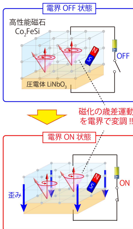
図 1. 本研究で実証したハーフメタル材料/圧電体界面マルチフェロイク構造(左)と磁化ダイナミクスの電界変調の概念図(右)。電界の制御(ON/OFF)で圧電体の結晶の歪みが磁性体中に伝搬することで、磁性体中の磁化ダイナミクス(磁化の歳差運動)が変調される。
