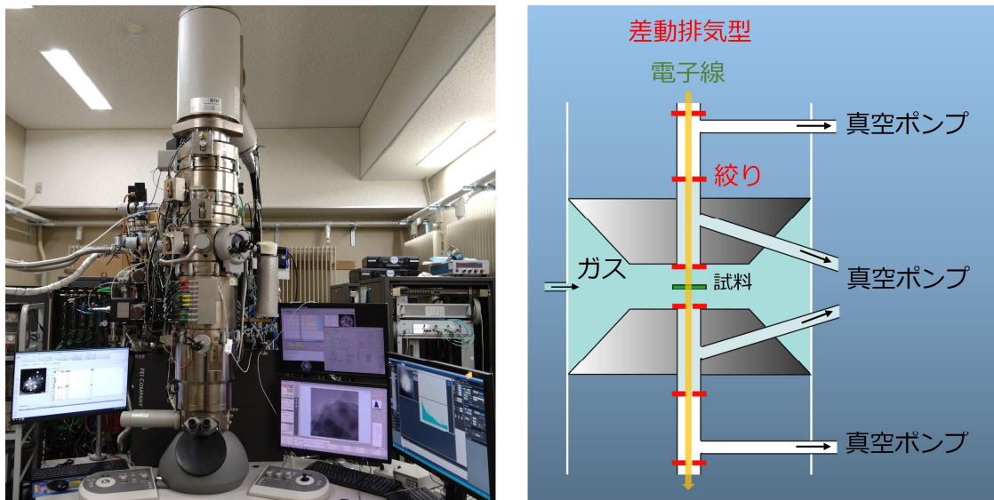
図1 環境制御型透過電子顕微鏡法 電子顕微鏡の外観図（左図）とガス導入機構の模式図（右図）。
