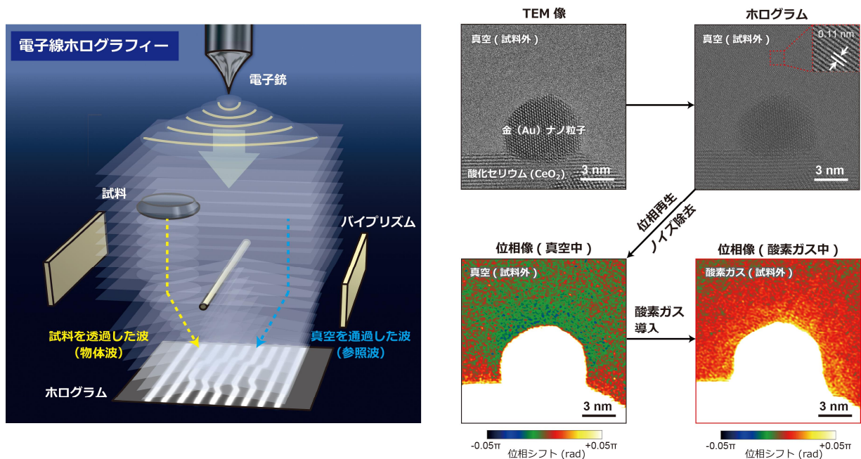
図2 高感度の電子線ホログラフィー 電子線ホログラフィーの模式図（左図）と電位分布に対する高精度解析の手順（右図）。
