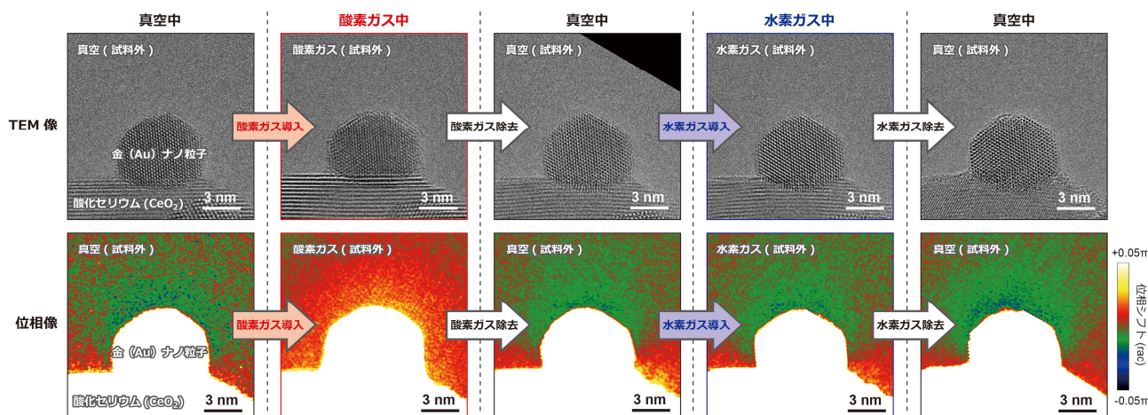
図3 様々なガス雰囲気中での触媒ナノ粒子の観察
