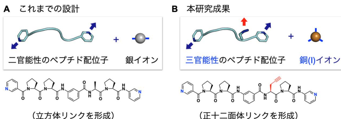
図2 分子設計 (A：以前の設計、B：今回の設計)
