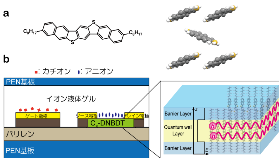
図1：有機半導体 C_8 -DNBDT の構造と電気2重層トランジスタの概略図
