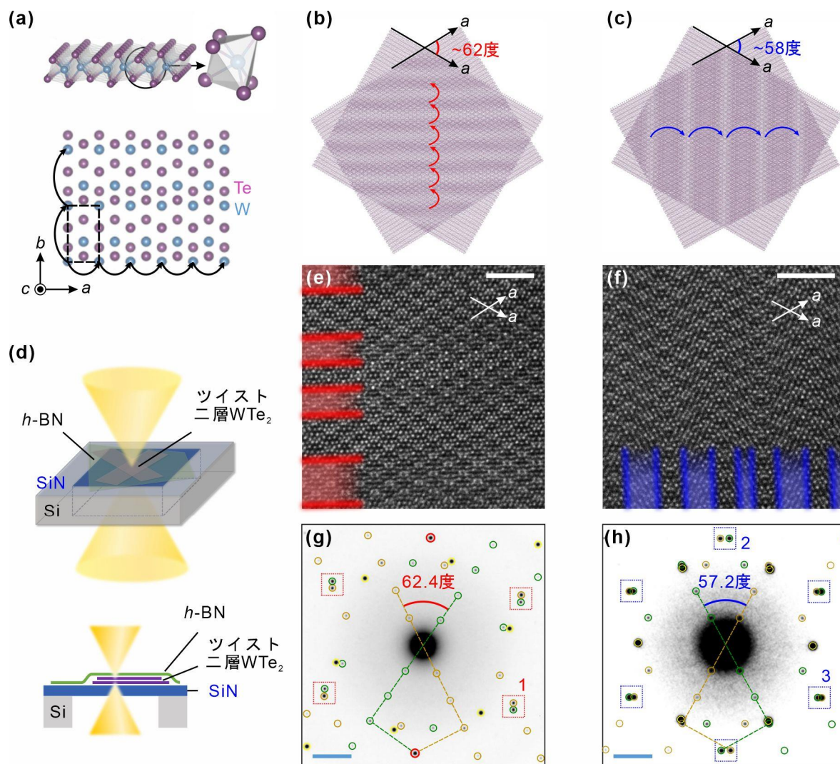
図 1：透過型電子線顕微鏡を用いたツイスト二層 \text{WTe}_2 の原子像観察。
