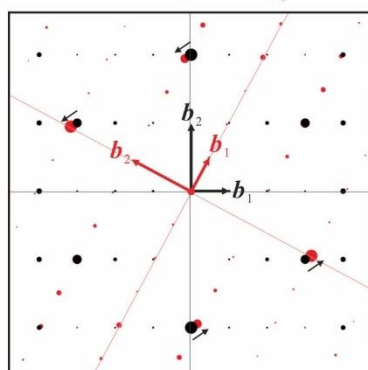
図 3：人工ツイスト二層 \text{WTe}_2 の電子回折パターンのシミュレーション。
