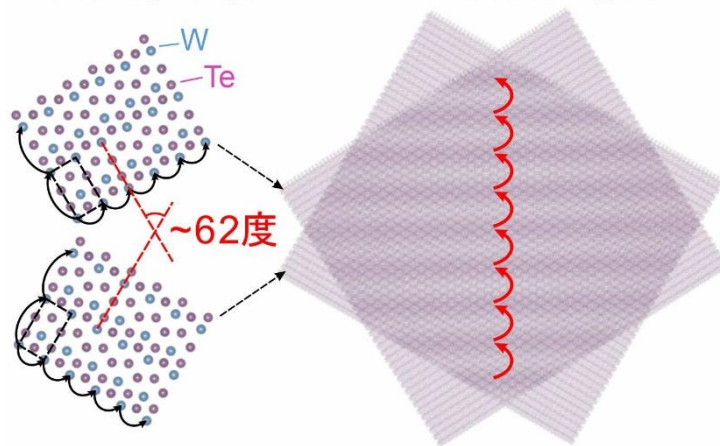
二次元原子層 \text{WTe}_2 のツイスト積層による一次元モアレ超格子の形成
