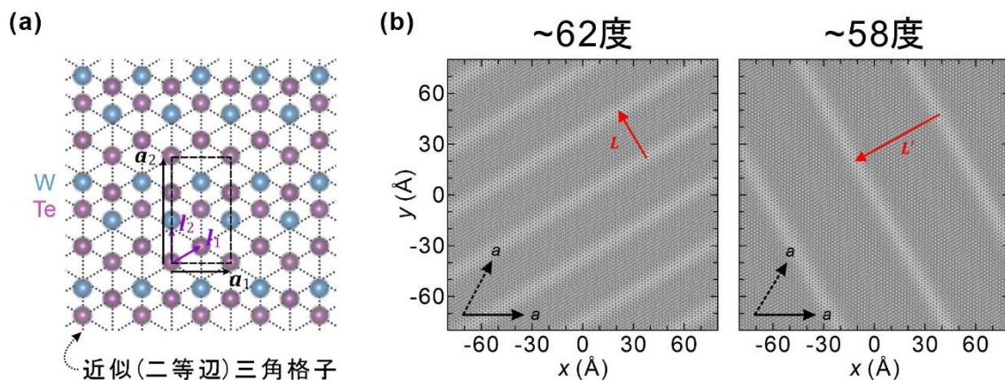
図 2：近似三角格子モデルを用いた一次元モアレ超格子の再現。
