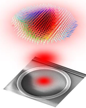
マイクロリング共振器による光スキルミオン生成
