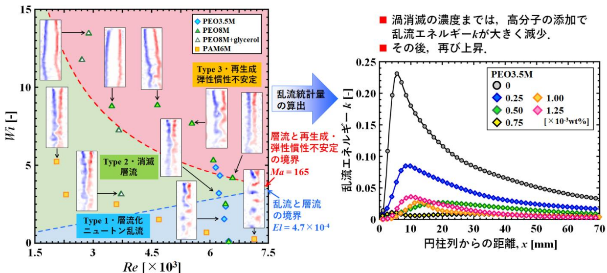
図 2: (左図) Re と Wi による渦放出の特徴の分類。 Ma は粘弾性マッハ数と呼ばれ、 Ma = \sqrt{Re/Wi} で表される無次元数。 El は弾性数と呼ばれ El = Wi/Re で表される無次元数。(右図)円柱下流の乱流エネルギー。高分子を添加すると、添加していない場合に比べ、乱流エネルギーは大きく低下する。渦が完全に消滅する PEO3.5M を 0.75 \times 10^{-3} wt% 添加した溶液まで、乱流エネルギーが低下し、渦が再生成する 1.00 \times 10^{-3} wt%、 1.25 \times 10^{-3} wt% で再び上昇した。
