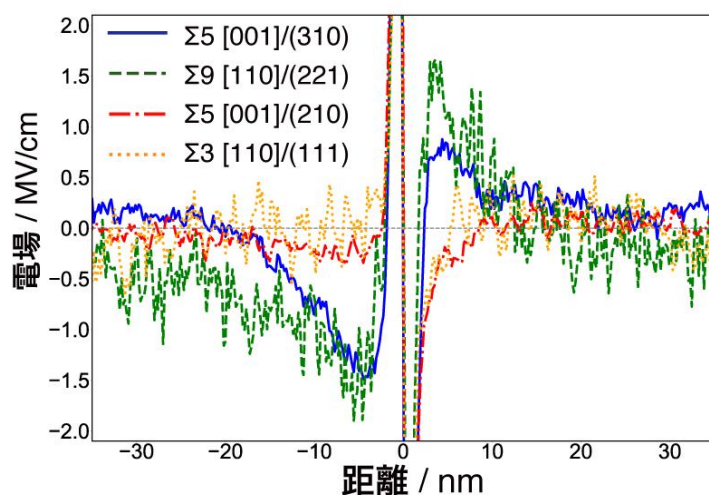
図4：今回観察した4つの結晶粒界における、水平方向電場の場所による分布。 イットリウムが多く偏析し高濃度化している2つの粒界 \Sigma 9 [110]/(221) （緑色）、 \Sigma 5 [001]/(310) （青色）において、空間電荷層の電場が大きく存在していることが分かる。一方、 \Sigma 5 [001]/(210) （赤色）、 \Sigma 3 [110]/(111) （橙色）では、電場も小さいことが分かる。
