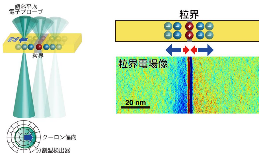
図1：本研究内容の概要。左がtDPC法による空間電荷層の電場観察の模式図。試料（黄色直方体、粒界を灰色部で示す）に対して、複数の角度で傾けた電子線（傾斜平均電子プローブ）をスキャン（図中では3箇所）し、透過した電子線を分割型検出器で検出する。
