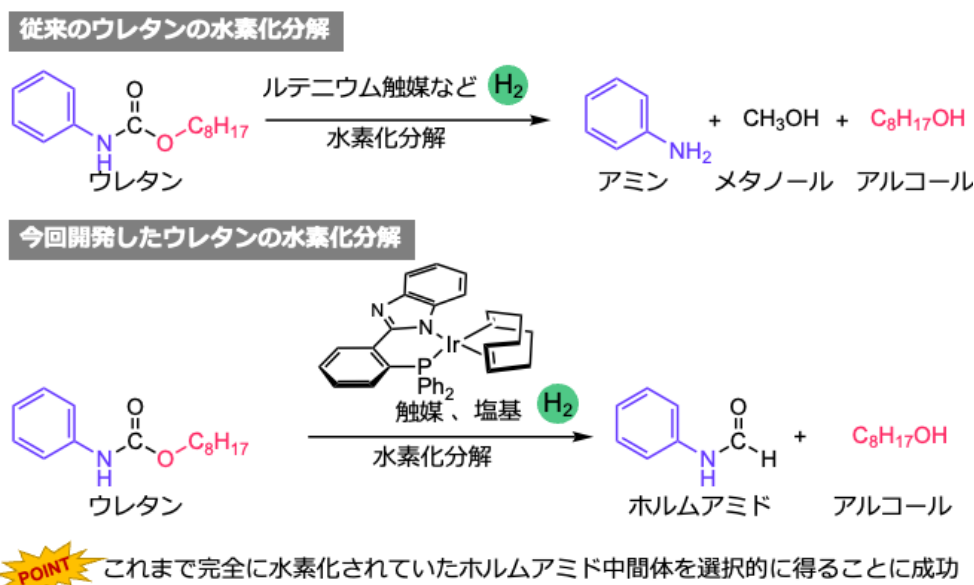
図 2：従来のウレタンの水素化分解と今回開発したウレタンの水素化分解
