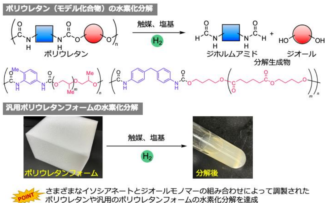
図4：ポリウレタンの水素化分解
