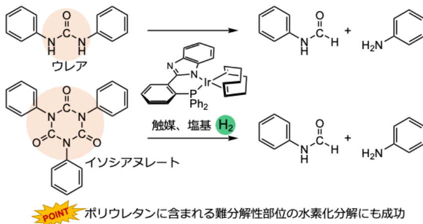
図 3：ポリウレタンに含まれる難分解性部位の水素化分解
