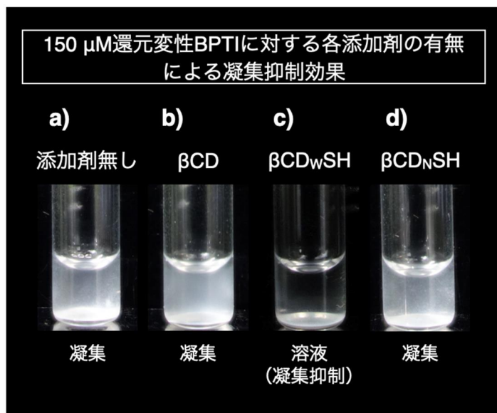
図 3 \beta CD W SH による還元変性 BPTI の高濃度条件での凝集抑制とフォールディング促進
