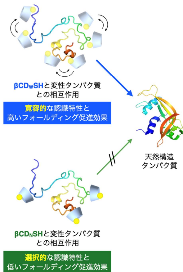
図 1 a) 「寛容的」な基質認識とタンパク質フォールディングの概念図、b) 本研究で開発した人工フォールディング促進酵素 \beta\text{CD}_w\text{SH} 、およびその比較分子 \beta\text{CD}_n\text{SH} の分子構造
