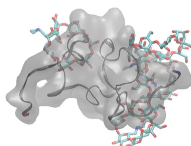
b) 還元 BPTI + \beta CD N SH
