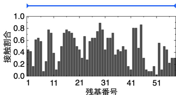
図 2 分子動力学シミュレーションの結果
