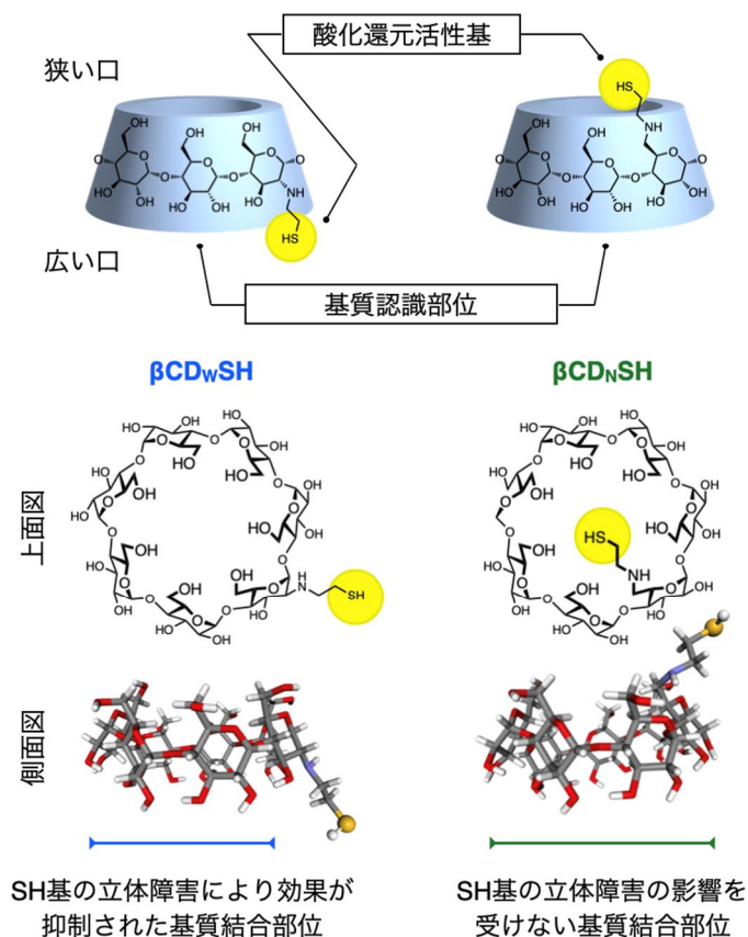
図 1 a) 「寛容的」な基質認識とタンパク質フォールディングの概念図、b) 本研究で開発した人工フォールディング促進酵素 \beta\text{CD}_w\text{SH} 、およびその比較分子 \beta\text{CD}_n\text{SH} の分子構造
