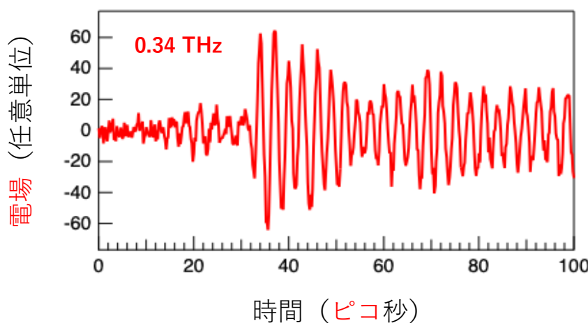
図1 半導体テラヘルツ発振器から放射されたテラヘルツ電磁波の振動電場波形。 数ピコ秒（1ピコ秒は0.000000000001秒）周期の超高速振動波形が変化する様子を捉えた。
