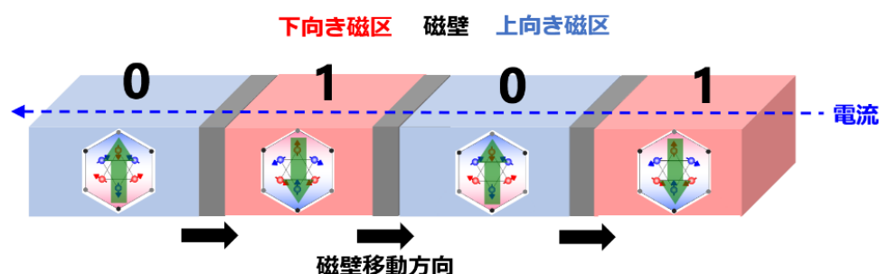
反強磁性体の磁壁移動による磁気シフトレジスタ（磁区の向きで“0”と“1”を記録）
