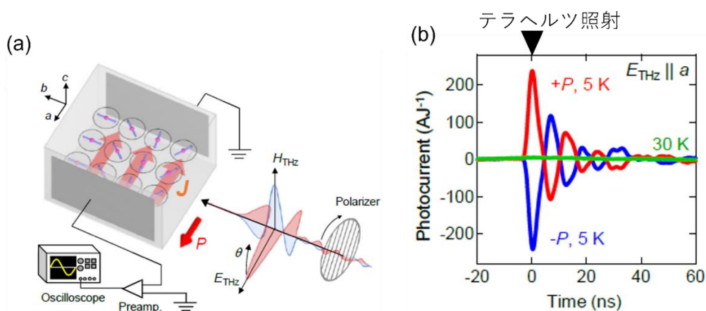
図1：(a)テラヘルツ光電流の測定の配置図。サンプル(灰色の直方体)にテラヘルツ光パルスを入射し、発生したa軸(極性方向)に平行な光電流を測定した。(b)得られた光電流の時間波形(縦軸は光電流、横軸は時間)。強誘電状態の5ケルビンにおいては、強誘電分極(P)の方向に従って光電流(J)が観測された(赤・青線)。今回テラヘルツ光パルスを照射しているため、光電流も瞬時的(ナノ秒、10億分の1秒の領域)に生成されている。一方で、常誘電状態の30ケルビンでは、光電流の信号が消失している(緑線)。
