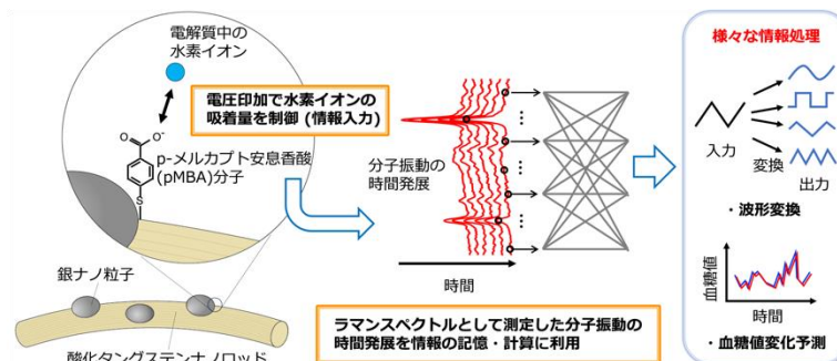
図：少数の有機分子（p-メルカプト安息香酸）の分子振動を用いる物理リザーバーコンピューティング
