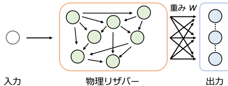
図1. 物理リザバーコンピューティングの模式図（本研究のように入力数が1の場合）。
