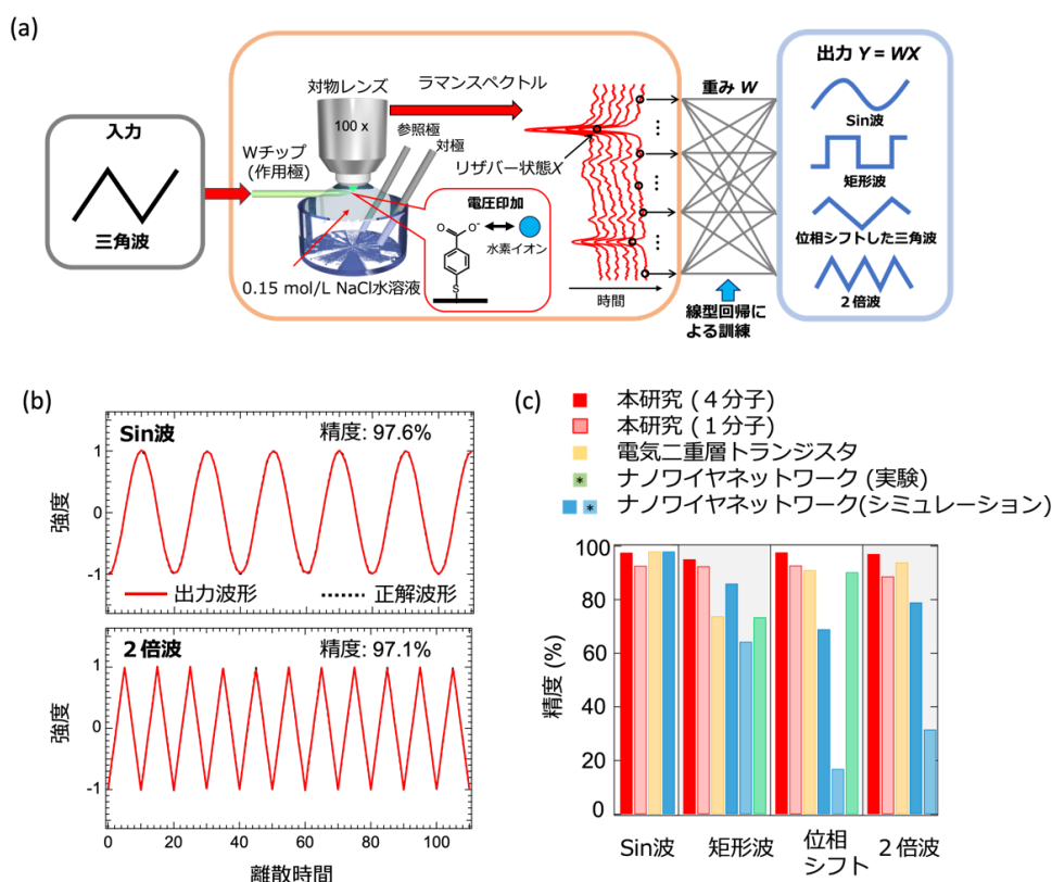
図 3. (a) 波形変換の模式図。 (b) Sin 波、および 2 倍波への変換を行った結果。 (c) 本研究と既報のデバイスとの性能比較。
