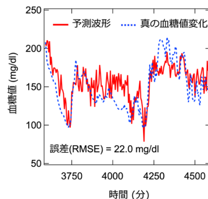
図 4. 血糖値変化を予測した結果と真の血糖値変化の比較。
