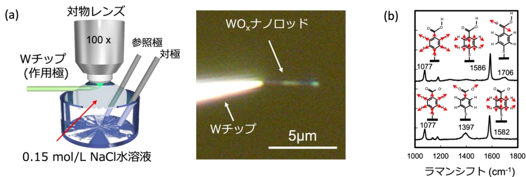
図2.(a) 本研究で用いた3端子型電気化学セルのイメージ図（左）。 \text{WO}_x ナノロッドおよび W チップの顕微鏡画像（右）。(b) 様々な分子振動モードを含む pMBA 分子のラマンスペクトル。（上段）水素イオンの吸着量が多い状態。（下段）水素イオンの吸着量が少ない状態。
