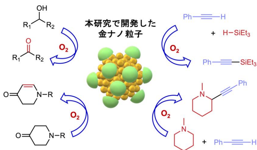
図 2：本研究で開発した金ナノ粒子による触媒反応
