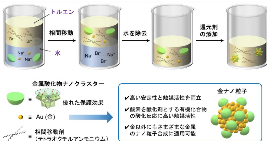
図1：安定性と反応性を両立した金ナノ粒子触媒の合成方法
