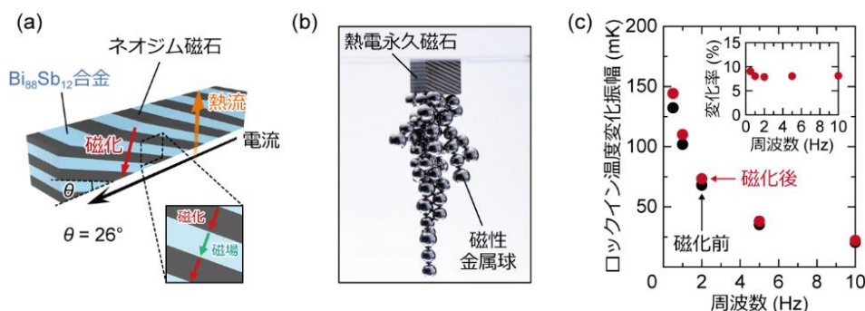
図4 永久磁石を組み込んだ人工傾斜型多層積層体(熱電永久磁石)における横型熱電変換
