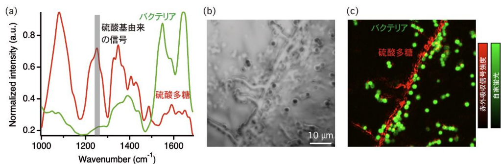
図2: バイオフィームマトリックス内の超解像赤外イメージングの結果
