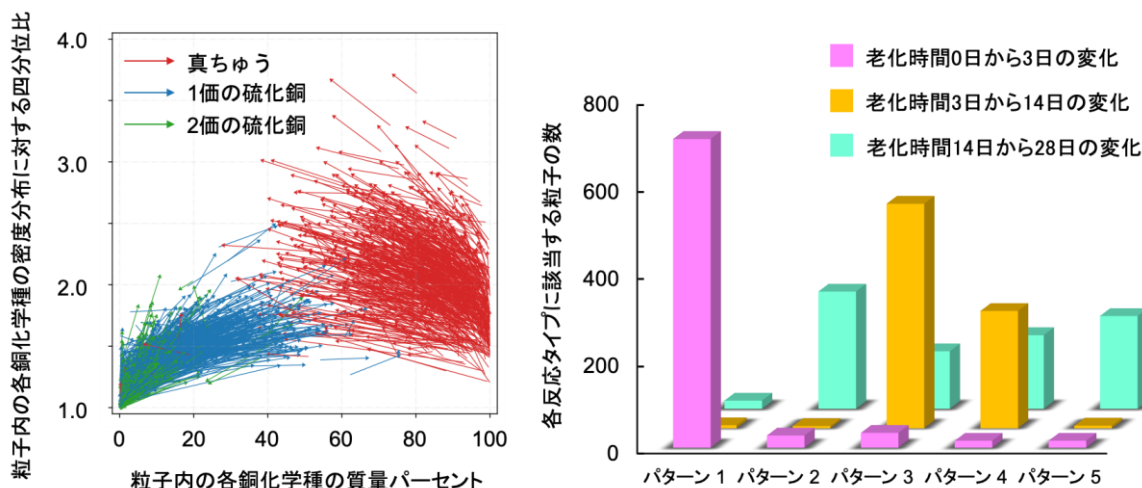
図 2. (左)可視化した 3 種類の銅の化学種について、湿熱老化に伴う化学種の反応の仕方やその度合いを矢印(ベクトル)を用いて視覚的に示した図。矢印の長さや方向が反応の違いを表している。(右)機械学習により分類された 5 種類の反応パターンの内訳を示した図。3 日目までの湿熱老化では、真ちゅうが硫化されて一価の硫化銅が生成するパターン1の反応が主であるのに対し、3-14 日までの湿熱老化では、パターン1は消失し、パターン3と4(2 価の硫化銅が生成する)が起こる。湿熱老化の最終段階(14-28 日)では複数の反応が並行して起こることがわかった。
