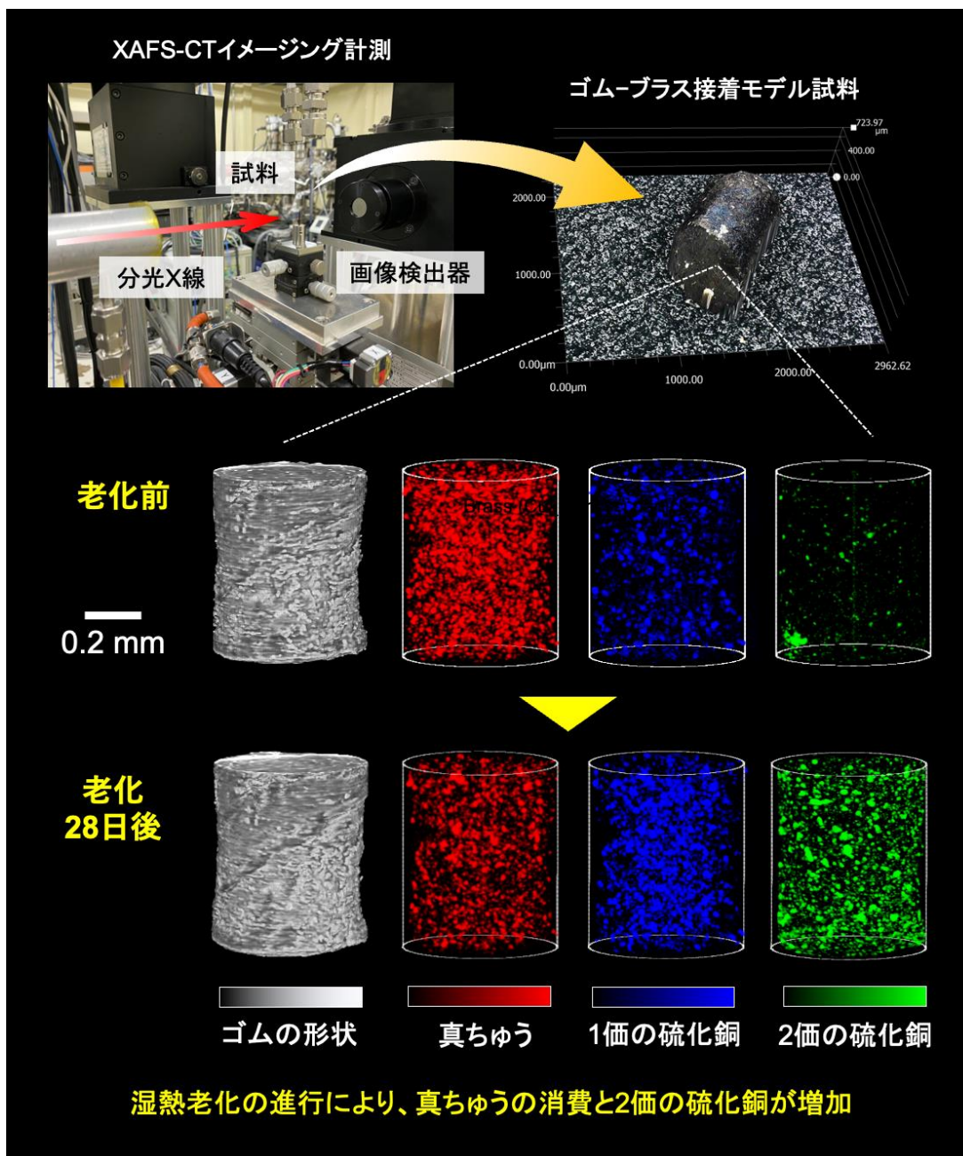
図 1. ゴムに真ちゅう粒子を混ぜ込んだ接着モデル材料に対する XAFS-CT イメージング。ゴム中に含まれる 3 種類の銅の化学種の分布と量を三次元的にイメージングし、湿熱老化反応による銅の状態の変化を非破壊で可視化することに初めて成功した。湿熱老化によって、真ちゅう成分(赤色)の消費が進み、2 価の硫化銅(緑色)が試料全体で生成していく様子が観察された。
