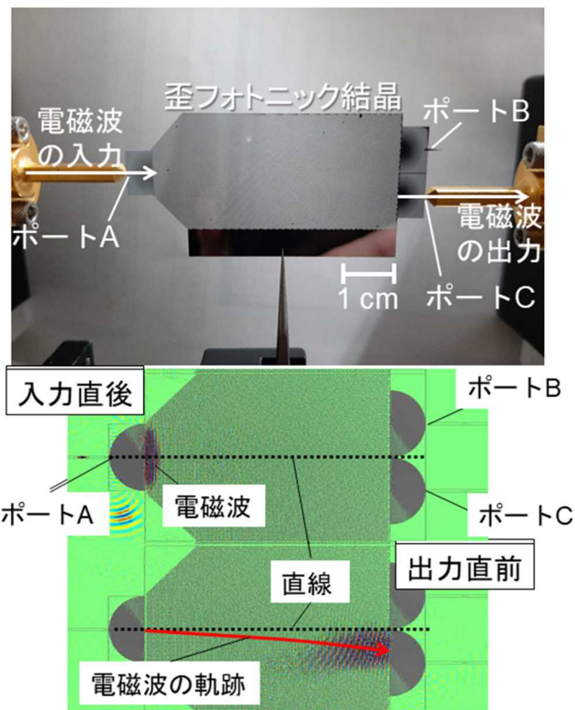
図 2. 実験の様子と歪フォトニック結晶における電磁波の伝搬のシミュレーション結果。ポート A から入った電磁波は真っ直ぐ進むとポート B と C に等価に入る。歪フォトニック結晶では、その伝搬方向が曲げられ、ポート C 側に伝搬する様子がわかる。
