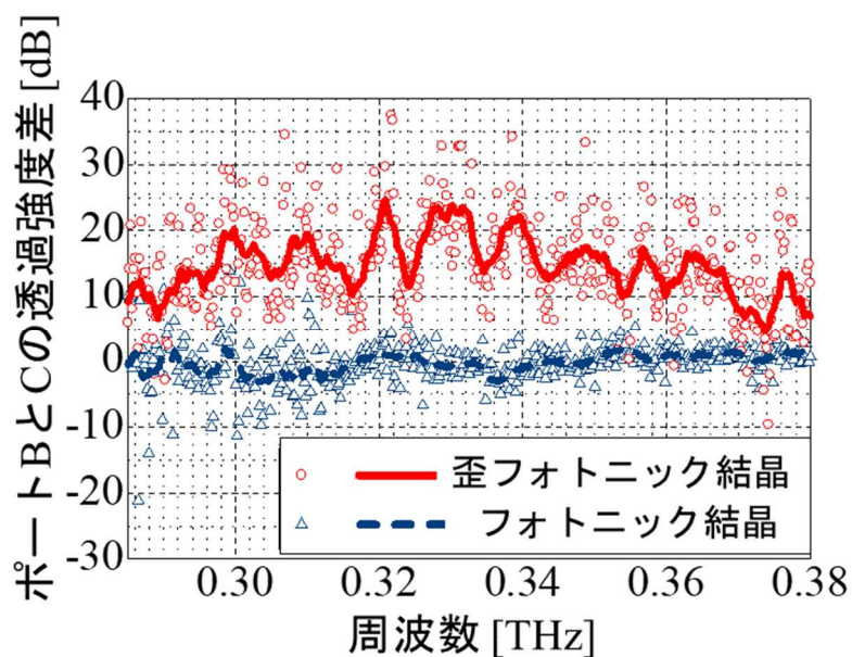
図 3. 実験結果。歪フォトニック結晶ではポート B と伝搬方向の曲げに対応するポート C での出力の強度差が得られた。
