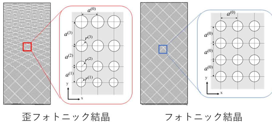
図 1. 歪フォトニック結晶と通常のフォトニック結晶の模式図。 a^{(0)} は正方格子フォトニック結晶における格子点の周期（格子定数）であり、歪フォトニック結晶ではその基本周期 a^{(0)} から、わずかに変化させる。平均的な誘電率を一定にするため、格子定数の変化に応じて、孔の大きさ r も変化させる。
