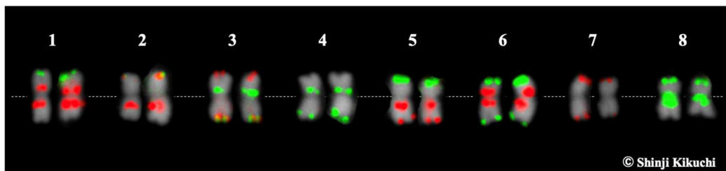
図1 DNAプローブを用いた染色体型分析 2色のDNAプローブを用いることにより、染色体塩基配列が実際の8本の染色体と一対一に対応していることが分かりました。
