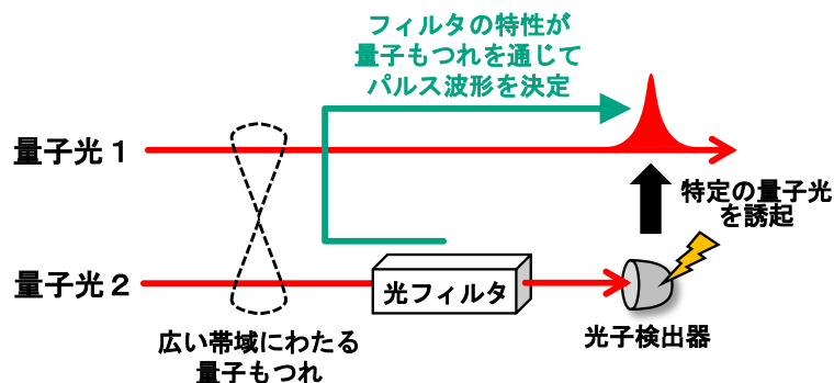
図2：量子光のパルス波形制御の原理
