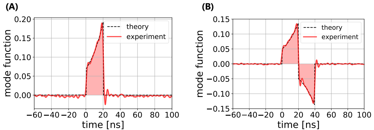
図3：生成したシュレディンガーの猫状態のパルス波形
