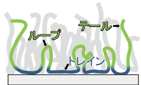
図1 トレイン・ループ・テールモデル
