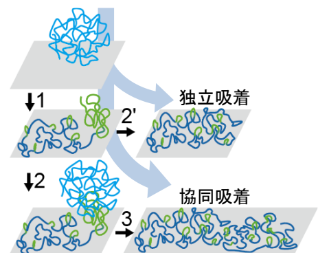
図3 固体界面における高分子吸着過程
