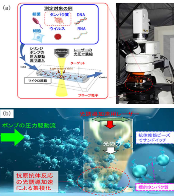
図1：(a) マイクロフロー光誘導加速システムの概略 (b) タンパク質を微量検出する原理のイメージ
