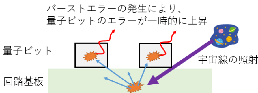
(図2) 宇宙線の照射によるエラー率上昇のメカニズム
