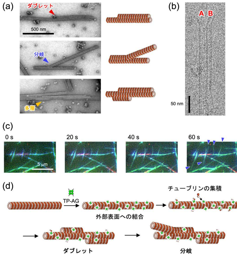
図 4. TP-AG の複合化による微小管超構造体の (a) ネガティブ染色電子顕微鏡像および (b) クライオ電子顕微鏡像。(c) 全反射照明蛍光顕微鏡による分岐構造の成長過程追跡。青矢頭は成長した分岐構造を表している。(d) ダブレットおよび分岐の推定形成メカニズム。
