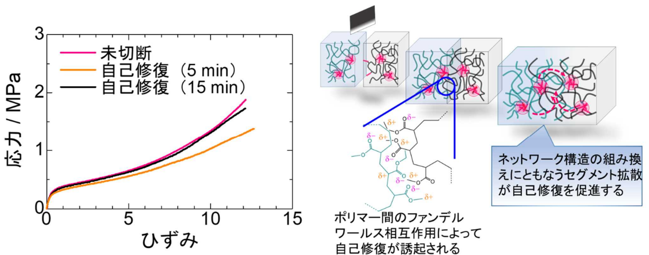
図2. 切断した PolyF が室温ですばやく自己修復する様子と、自己修復メカニズムの概略図。この様な迅速な自己修復は、ポリマー同士の分子間相互作用が強いことに起因する。
