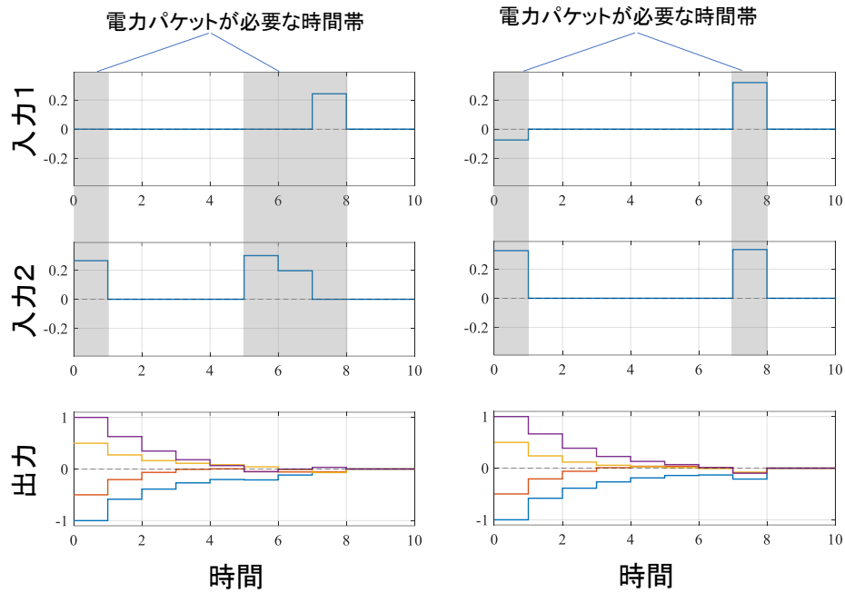
図 2：従来法（スパース制御）（左図）と今回の方法（右図）を適用したときの制御入力と状態の応答の例。従来法の場合、2つのアクチュエータが同時に休止する時間帯が短い（電力パケットが必要な時間帯が長い）が、開発した方法では、同時に休止する時間帯が長い。
