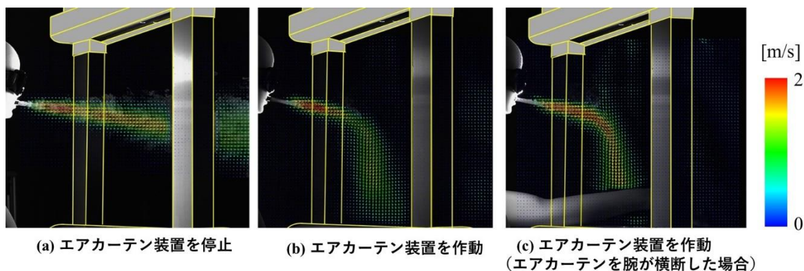
図4: 呼気から発するエアロゾルの遮断効果の検証（粒子画像流速測定法による可視化結果） (a) エアカーテン装置を停止、(b) エアカーテン装置を作動、(c) エアカーテン装置を作動 (エアカーテンを腕が横断した場合)
