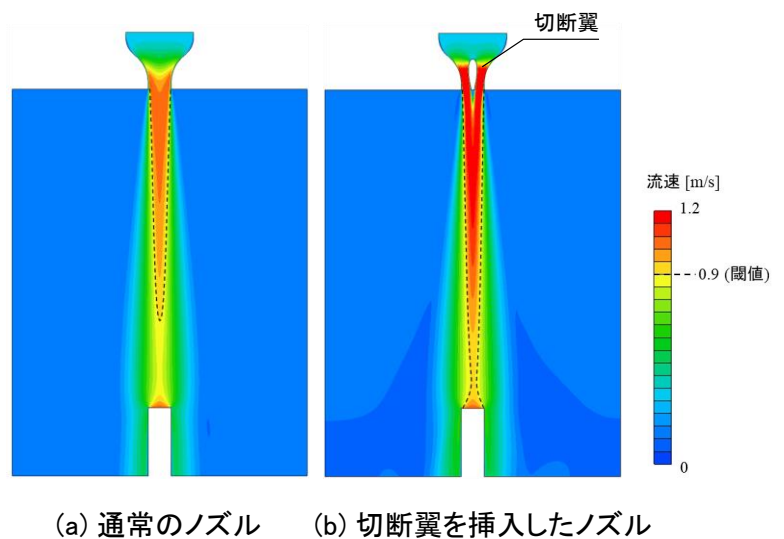
図 3: エアカーテン気流の平均速度ベクトル。 (a) 通常のノズル (b) 切断翼を挿入したノズル
