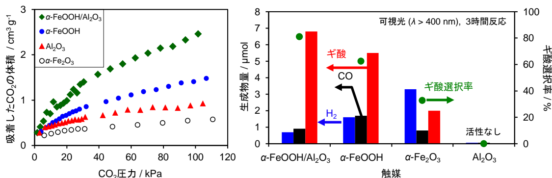
図 2. 様々な触媒試料の CO 2 吸着能力(左)と CO 2 還元活性比較(右)
