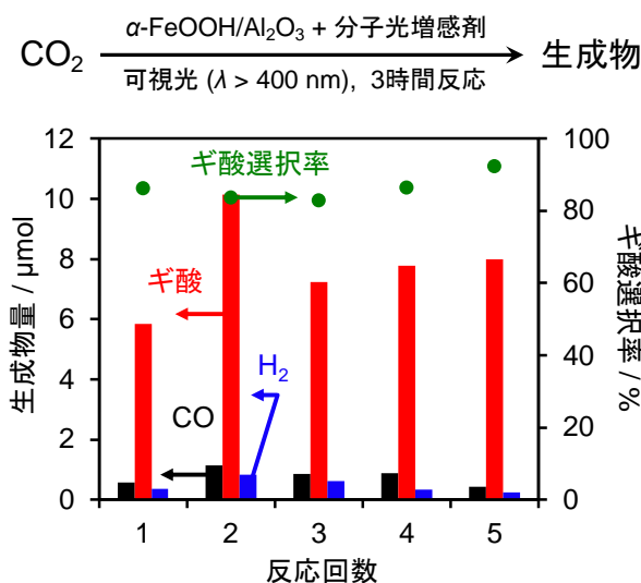
図1. α-FeOOH/Al 2 O 3 触媒によるCO 2 還元反応（繰り返し反応試験）
