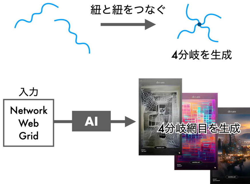
図 1： 紐と紐をつなぐと、自然に 4 分岐網目が形成される。また、AI 画像生成アプリ (Dream by Wombo) に network、grid、web などと網目構造を想起させるキーワードを与えると、ほぼ 4 分岐網目構造の絵が生成される。AI は基本的には、与えられたデータセット (すなわち人により書かれてきた膨大な絵の集合) の内部での推論を行うため、「網目といえば 4 分岐構造」が一般的であると推定される。
