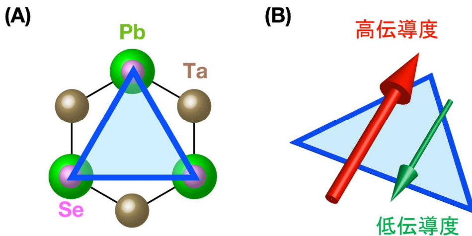
図1. (A) \text{PbTaSe}_2 の結晶構造の模式図(上面図)。3回回転対称性を有する空間反転対称性の破れた構造を持つ。 (B) 3回回転対称性を有する物質での整流現象の模式図。
