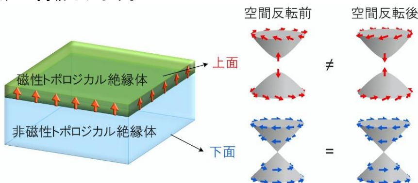
積層構造（左）と磁性トポロジカル絶縁体表面に生じるパリティ異常
