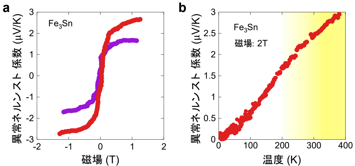
図 2 : カゴメ格子強磁性体 \text{Fe}_3\text{Sn} における磁気熱電効果
