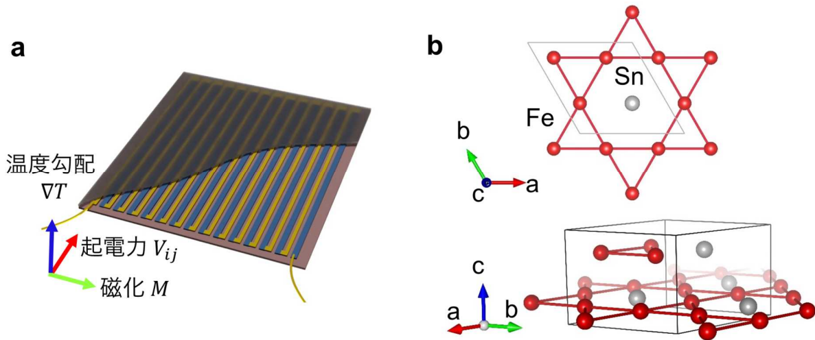
図 1 : 磁気熱電効果を活用した熱電変換モジュールと \text{Fe}_3\text{Sn} の結晶構造の概念図
