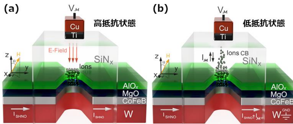
図2) 実験で明らかになった動作原理の説明図。(a)メモristaが高抵抗状態の場合は、上部電極に電圧( V_M )を印加すると、メモrista部分には電界が発生する。これによってCoFeB層に蓄積される電荷量に変化し、磁気特性が変調される。(b)メモristaが低抵抗状態の場合は、メモristaにはイオンの橋(Conduction Bridge)が形成され、上部電極に電圧( V_M )を印加すると、W/CoFeB 層へと電流が流れる。またこの橋の電気抵抗はアナログ的に変えられる。よって、
