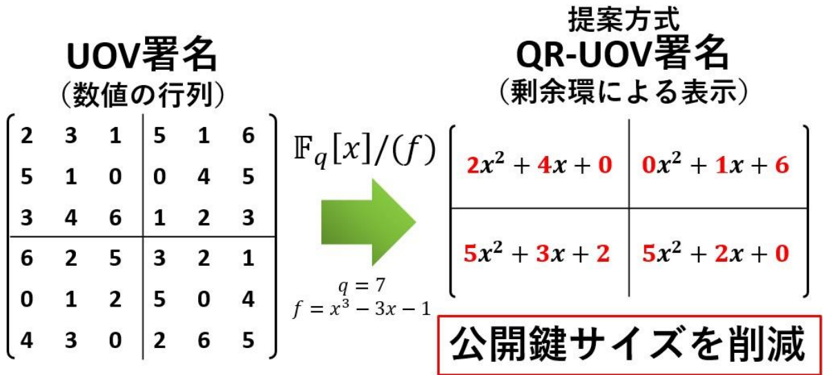
図 1. 提案方式の剰余環による公開鍵データサイズの削減
