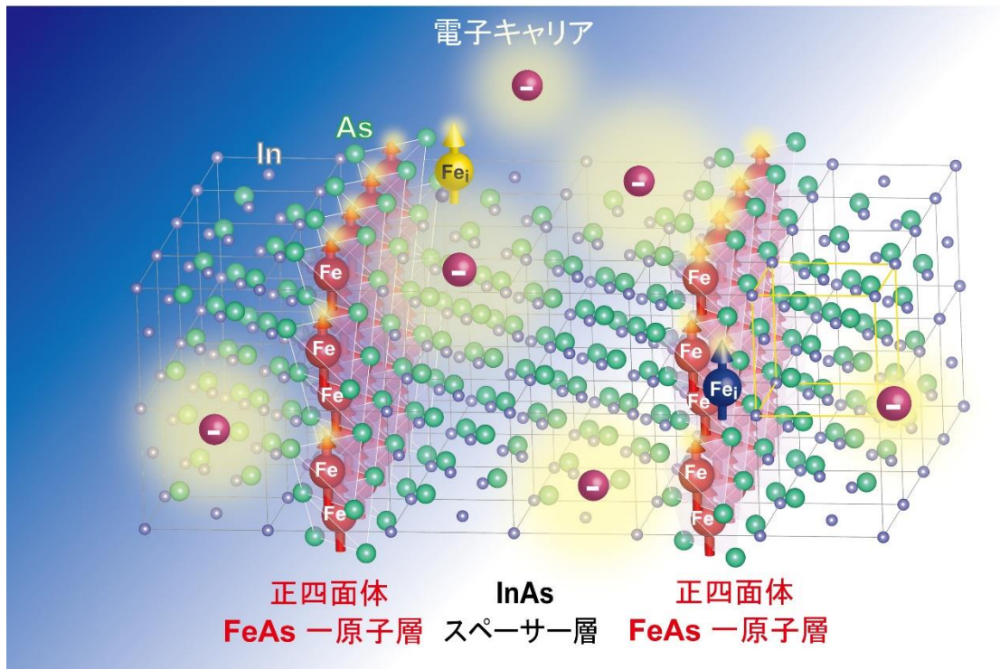
図1 本研究グループが作製した試料の構造：低温分子線エピタキシー結晶成長法による結晶成長を用いて InAs の閃亜鉛鉱型結晶構造（図中右上の黄色い枠で表した単位セルが繰り返した構造）を保ちながら Fe-As 正四面体結合を 1 原子層の平面内（ピンク色）に閉じ込めることに初めて成功した。この技術により、FeAs 原子層を InAs 結晶中に等間隔に埋め込む構造を作製し、世界初の単結晶 FeAs/InAs 超格子構造の作製に成功した。FeAs 原子層の間に超格子構造中に存在する電子キャリア（赤玉と黄色い雲＝電子の波動関数）を介した Ruderman-Kittel-Kasuya-Yosida (RKKY) 型の相互作用が働き強磁性秩序を成立させると考えられる。さらに、FeAs 原子層内の一部の Fe が格子間位置（黄色い Fe 原子）とアンチサイト位置（青い Fe 原子）にも存在し、FeAs 原子層のすべてのスピン方向を揃え強磁性を得るために重要な役割を果たすことを明らかにした。（図面の一部は VESTA より作製された）。
