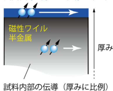
図1. 磁性ワイル半金属の表面伝導。
